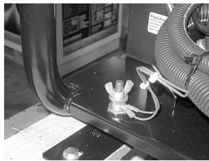
Figura 3-1. Conexión a tierra del generador
