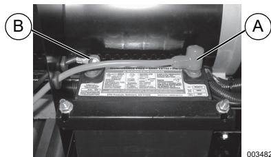
Figura 2-11. Conexión de la batería
