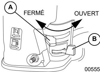
Figure 3-2. Robinet de carburant et étrangleur
