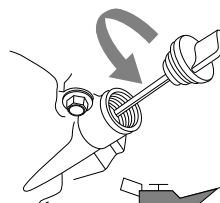
000115 Figure 4-5. Remplissage d'huile moteur
